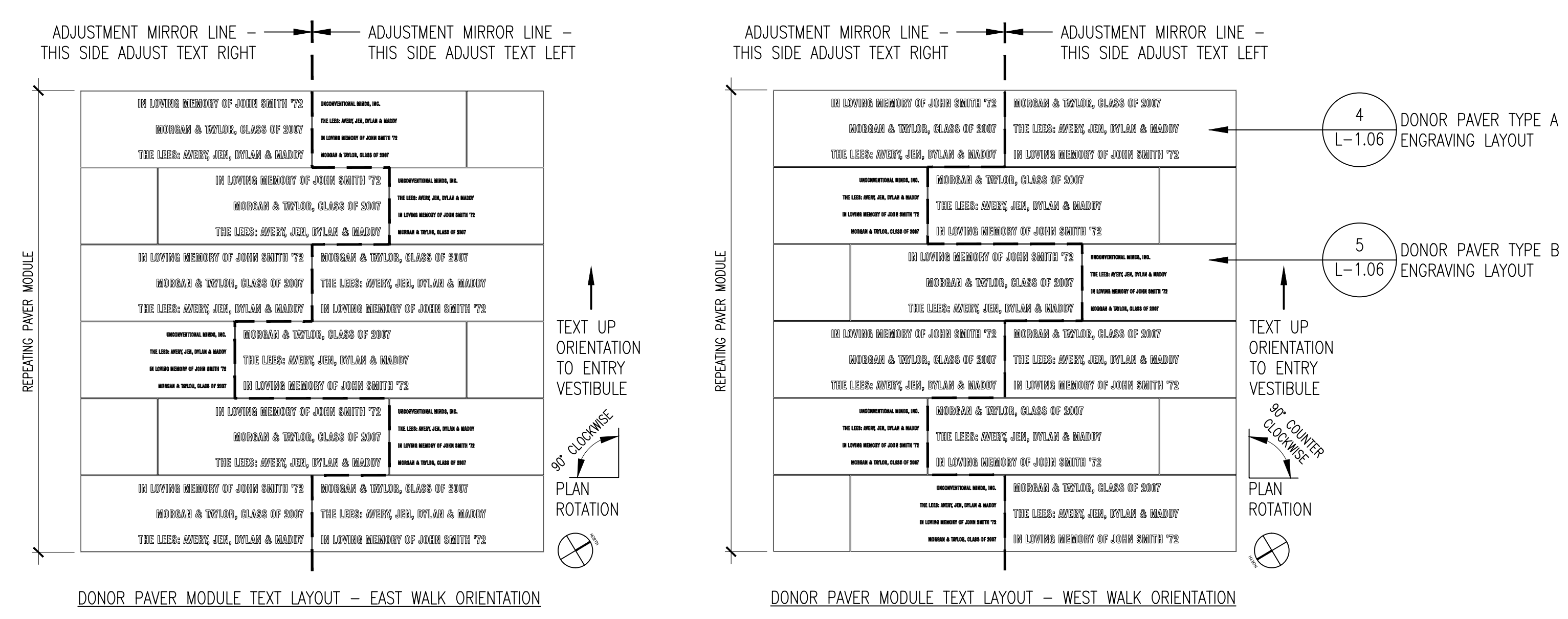
3 DONOR PAVER MODULE TEXT LAYOUT L1.06 SCALE: 1/2" = 1'-0"
